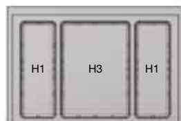
Cajón 800 Ancho 700 a 740 Fondo 430 a 490 Hueco tipo H1 + H3 + H1
