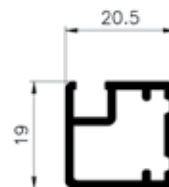
CUBIC - Perfil de 20,5 x 19 mm. en radio 1,5 Aluminio
