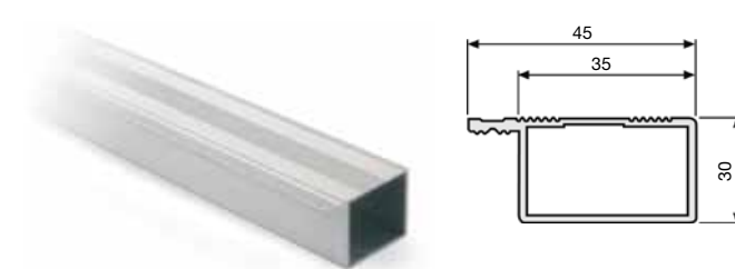
Perfil posterior de 30 mm. de 4,2 mts. Aluminio
