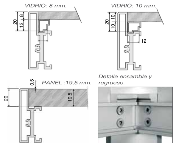
Instalación con diferentes gruesos de sobre:
