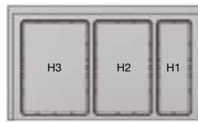
Cajón 900 Ancho 800 a 840 Fondo 430 a 490 Hueco tipo H3 + H2 + H1
