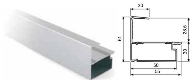
Perfil frontal de 30 a 60 mm. de 4,2 mts. Aluminio
