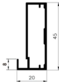
MINIM 8 - Perfil de 45 x 20 mm. pestaña de 8 mm. Aluminio
