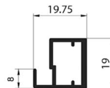
CUBIC REDUCIDO - Perfil de 19,75 x 19 mm. Aluminio
