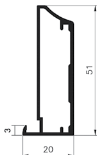
ELICA - Perfil de 51 x 20 mm. pestaña de 3 mm. Aluminio
